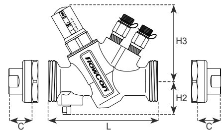
FlowCon ABV mit E-JUST-Kartusche
