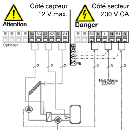
Fig. 3.2.7: Solaire avec échangeur thermique ext.
