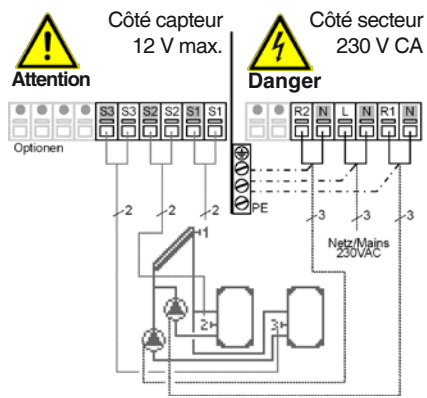
Fig. 3.2.11: Solaire 2 accumulateurs/2 Po.
