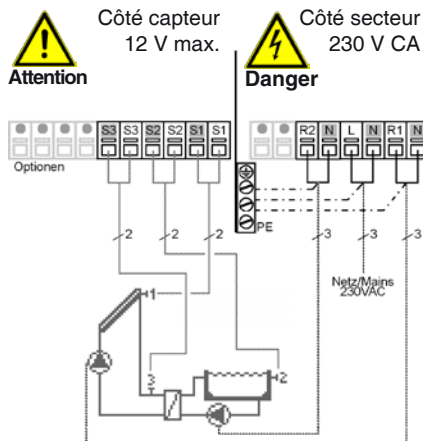
Fig. 3.2.13: Solaire avec piscine
