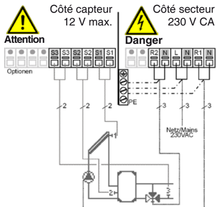
Fig. 3.2.5: Solaire avec augmentation ret.
