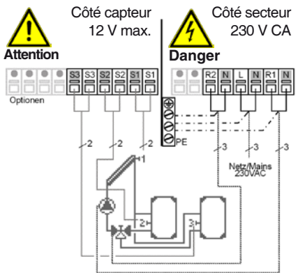
Fig. 3.2.10: Solaire 2 accumulateurs/vanne
