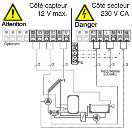
Fig. 3.2.14: Solaire Accumulateur/Piscine
