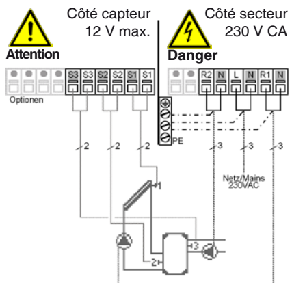
Fig. 3.2.3: Solaire + Thermostat
