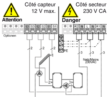
Fig. 3.2.12: Solaire avec accumulateur supplémentaire
