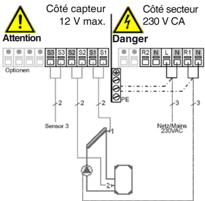
Fig. 3.2.2: Solaire avec accumulateur
