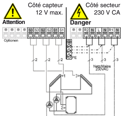
Fig. 3.2.9: Solaire 2 coll. 2 pompes
