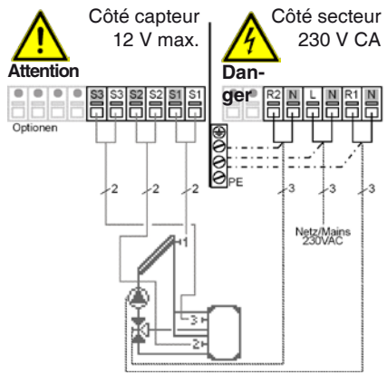
Fig. 3.2.6: Solaire avec accumulateur bi-zone
