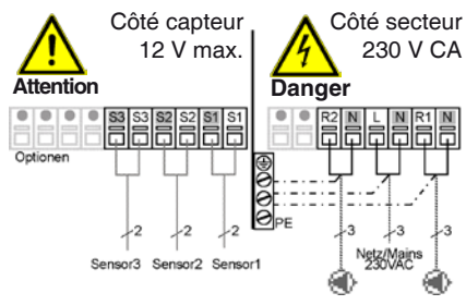
Fig. 3.2.15: Régulateur ΔT universel
