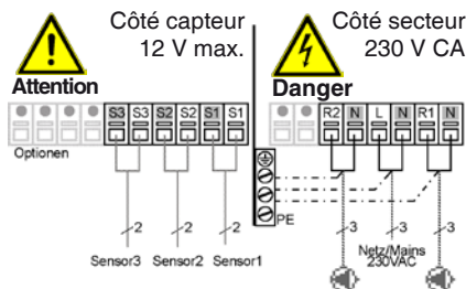
Fig. 3.2.16: Régulateur universel 2x \Delta T
