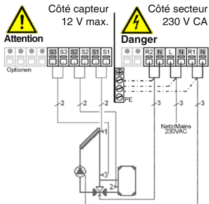
Fig. 3.2.4: Solaire avec dérivation
