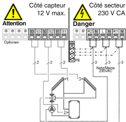
Fig. 3.2.8: Solaire 2 coll. (est/ouest)
